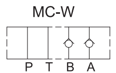
A 與 B 迴路控制 ( A & B Port )
